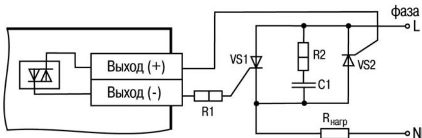
Рисунок Б.12 – Схема подключения нагрузки к ВЭ типа «С» двух тиристорных, подключенных встречно-параллельно ( R_2=47... 68 \text{ Ом} , C_1=0.1 \text{ мкф} \times 630 \text{ В} )
